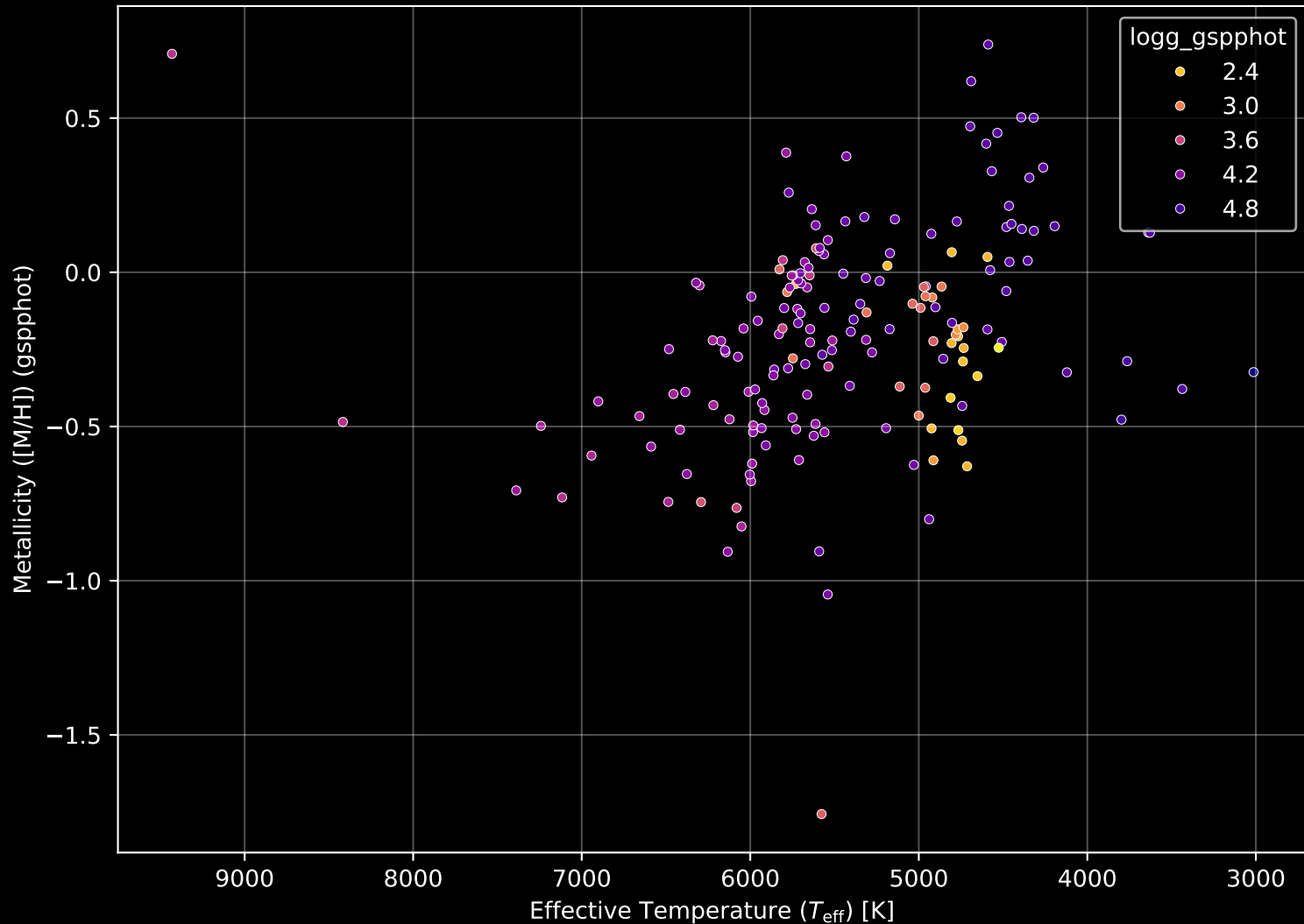
APOGEE DR17 Field: [187+48_MGA] Stellar Population Parameters (n= 176)
